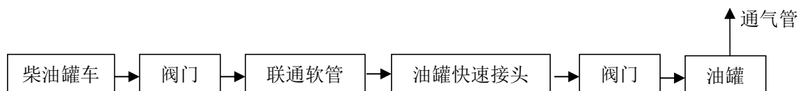
图 2-4 柴油卸油工艺流程方块图
