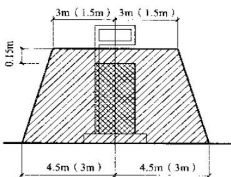
图 C.0.5 汽油加油机爆炸危险区域划分
