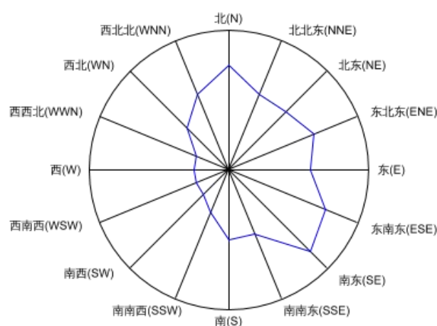
图 8-4 风向玫瑰图
