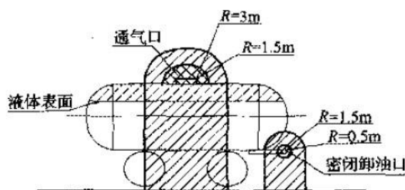
图 C.0.4 汽油的地面油罐、油罐车和密闭卸油口
