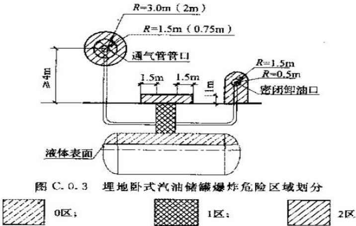
图 8-1 汽油罐爆炸区域图
