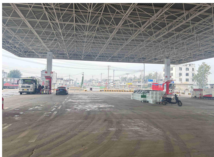
图 2-7 加油站加油区照片
