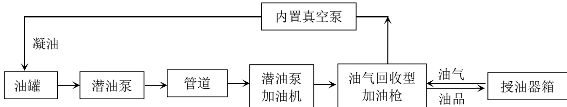
图 2-1 汽油加油工艺方块图（潜油泵）
